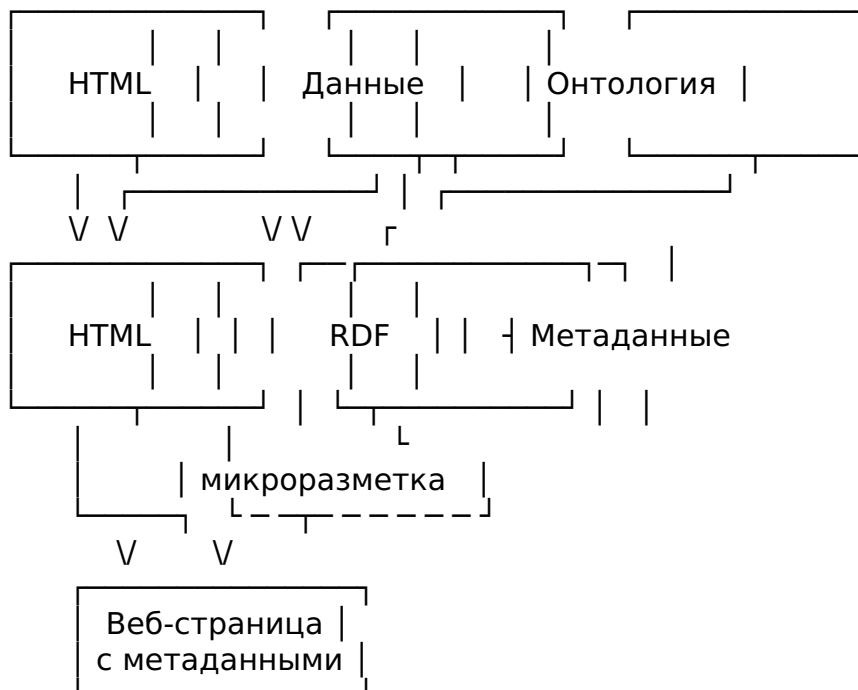
Рисунок 4 - Системное видение связей между метаданными, данными и онтологиями на примере открытых данных в RDF
