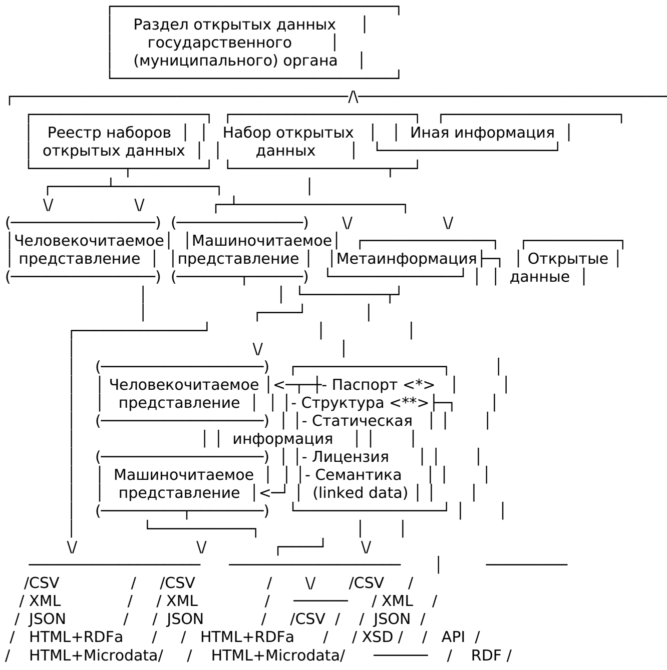
Рисунок 1 - Архитектура раздела открытых данных
